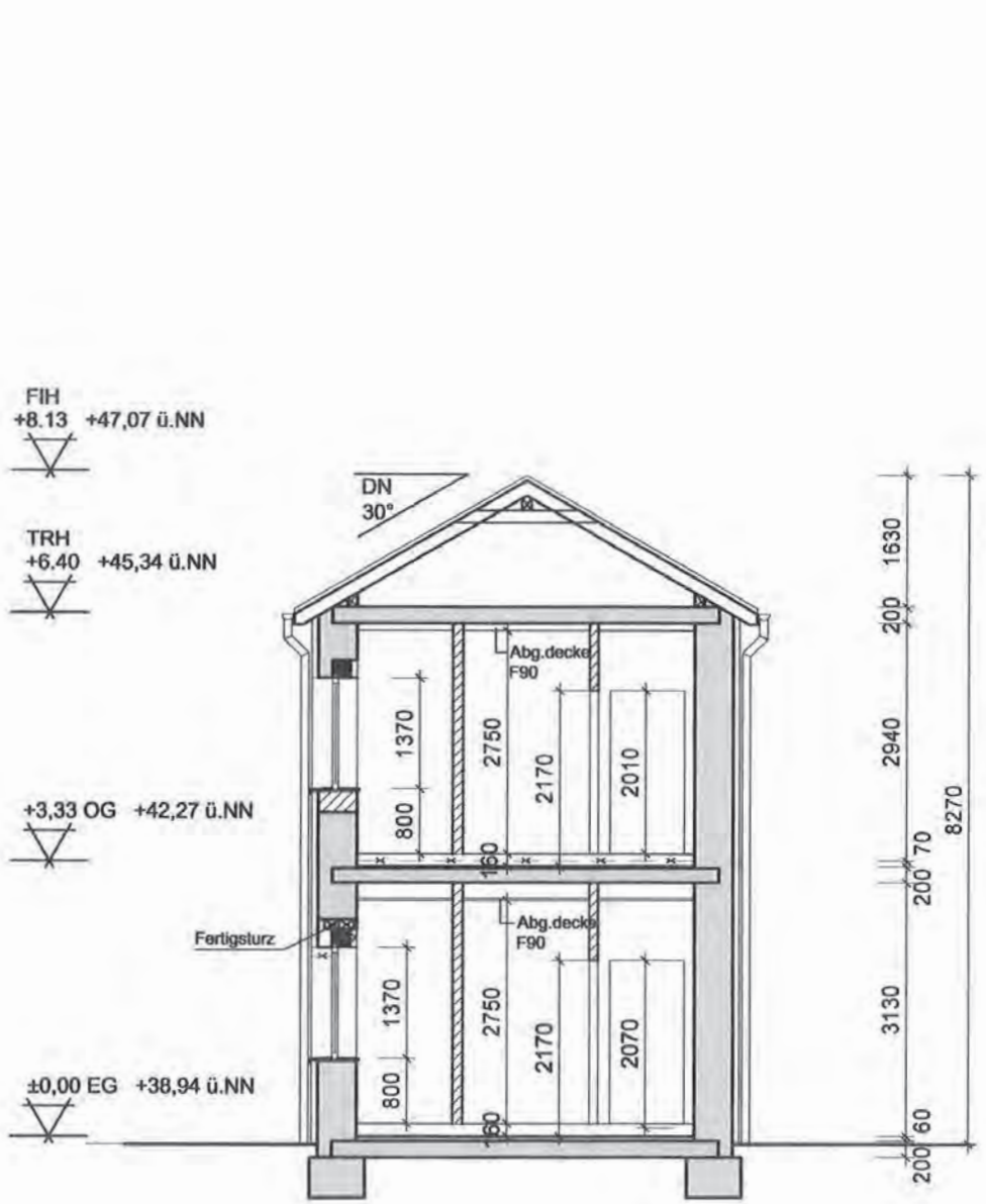
Schnitt B-B
