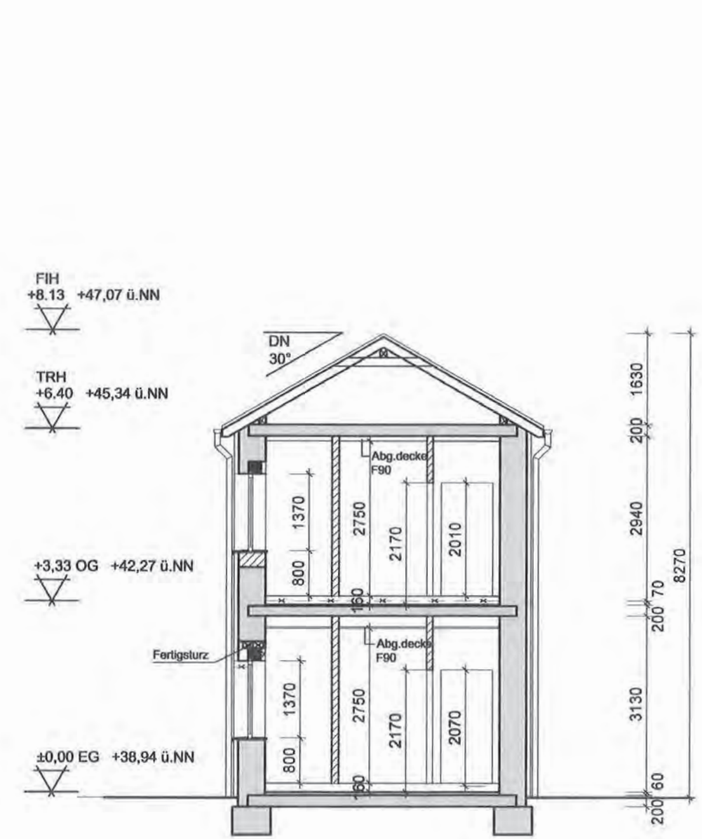
Schnitt B-B
